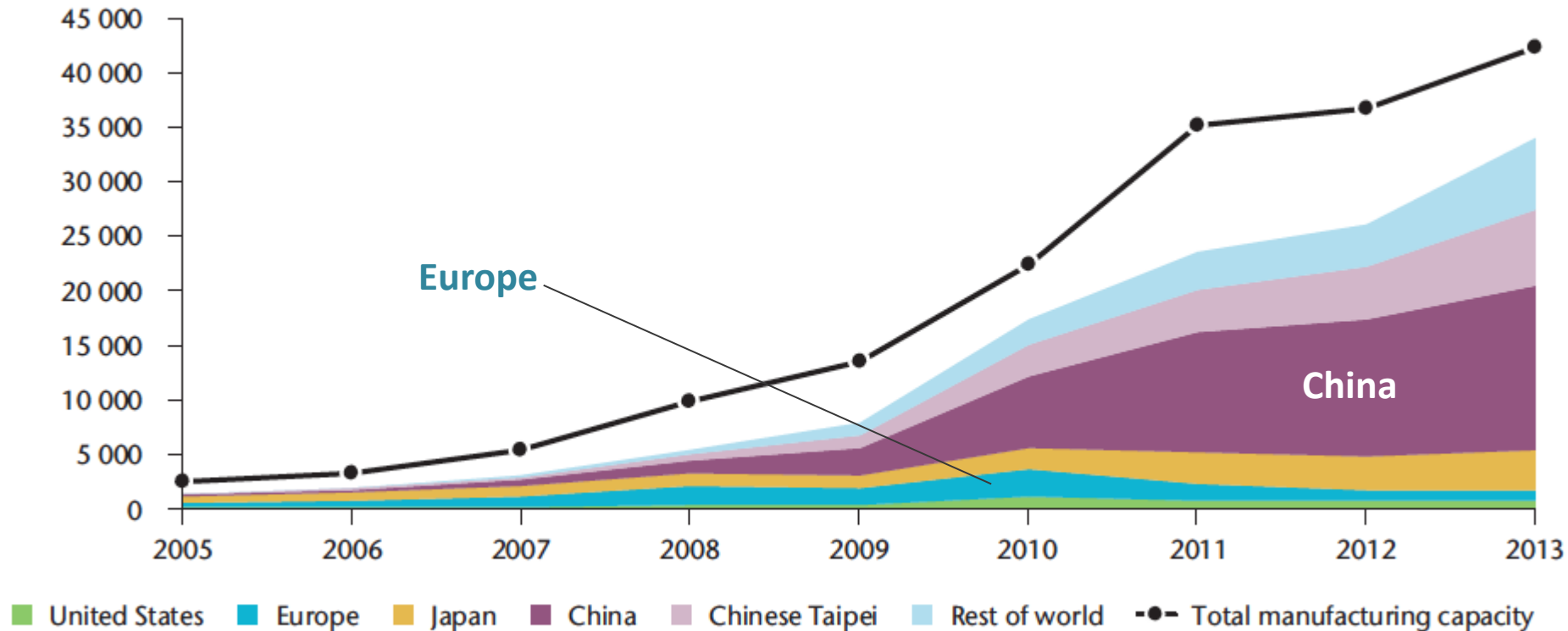
Fabrication de panneaux PV par pays [MW]
